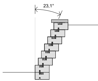
Odklon stěny o 23,1°, tj. 0,4m/1bm výšky.
