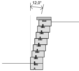
Odklon stěny o 12°, tj. 0,2m/1bm výšky.
